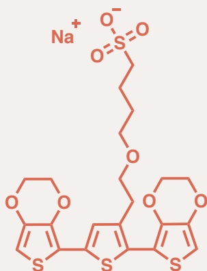
ETE-S Trimer
